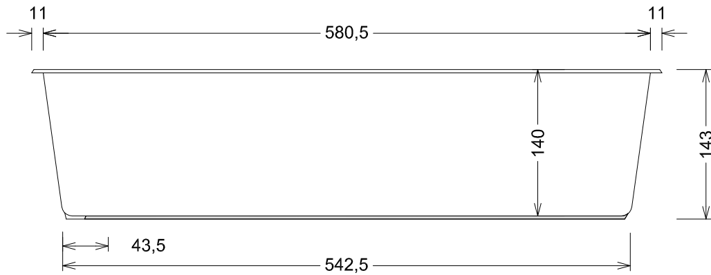
Schnitt - Section A - A
