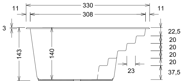
Schnitt - Section B - B
