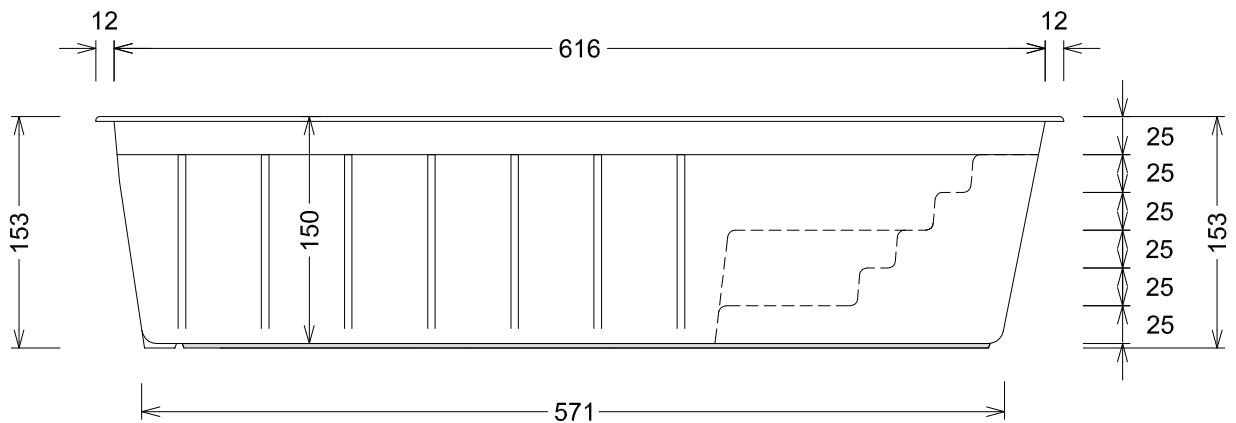
Seitenansicht - Side view
