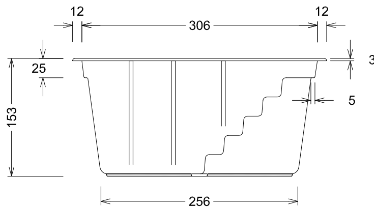
Ansicht Treppenseite - View stair side
